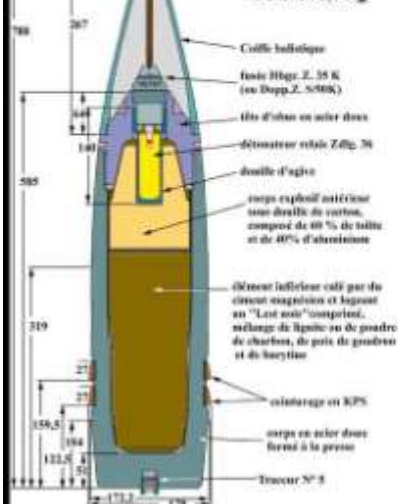
Obus explosif type 38 L.S. à coiffe balistique pour canon de 17 cm 17 cm K. Gr. 38 (Hb)(L.S.) Poids : 62,8 Kg
