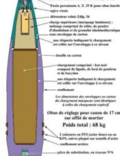
Obus de 17 cm type 39 L.S. (marqueur d'impact, à fusée AZ 35 K) 17 cm K. Gr. 39 L. S. m. A. Z. 35 K
