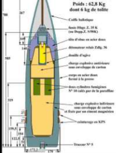
Obus explosif type 38 à coiffe balistique pour canon de 17 cm 17 cm K. Gr. 38 (Hb)
