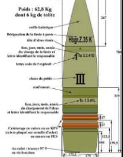
Obus explosif type 38 à coiffe balistique pour canon de 17 cm 17 cm K. Gr. 38 (Hb)
