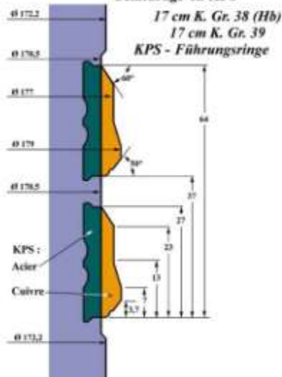
Obus explosif coiffé de 17 cm type 38 Obus explosif de 17 cm type 39 Ceinturage en KPS
